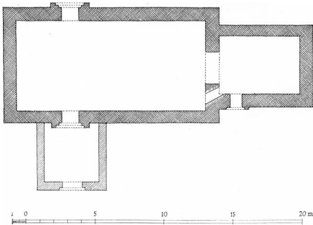
Fig. 2. Danmøre. Plan. 1:300. Målt af Aage H. Mathiesen 1885.
