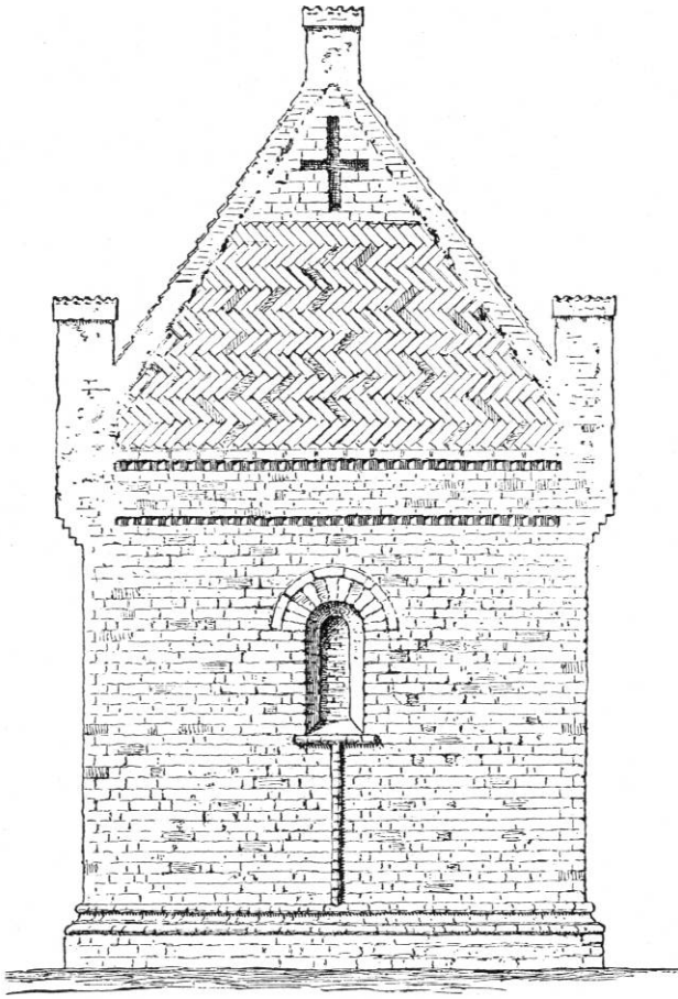
Fig. 3. Danmæse. Korgavl. 1:100. Efter tegning af Magnus-Petersen 1877.
