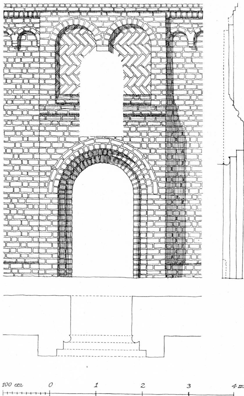
Fig. 4. Danmarch. Sydportal. 1:50. Målt 1896 af Magnus-Petersen. Rettet af Aage Roussell 1949.
